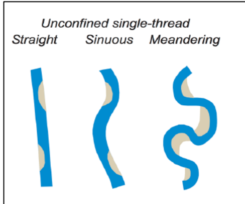
Obr. 5: Geomorfologické typy vodních toků podle půdorysných tvarů koryta (Just, 2005)
