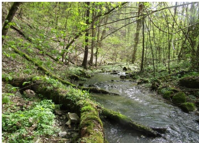
Obr. 14b: Další příklady erozních údolí typu V, zpravidla na horních úsecích toků, ale také v členitých terénech na středních tocích (přirozeně bez vyvinuté nivy, bez předpokladu posuzování rozlivu a dalších charakteristik); také v těchto příkladech břehová eroze odpovídá říčnímu vzoru (hydromorfologickému typu vodního toku) – viz parametr 5
