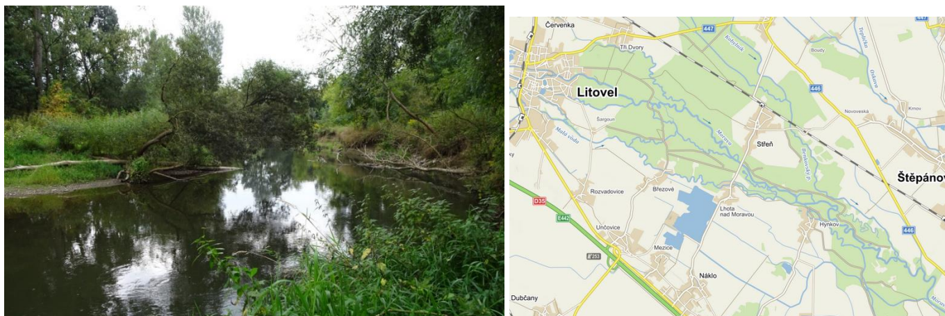
Obr. 11: V málo sklonitých pasážích říčních údolí nízkých poloh s širokou nivou vyplněnou hlubšími vrstvami aluviálního materiálu může být formován typ vodního toku se stabilně se větvcím korytem (anastomozní vodní tok) . Výrazně rozvinutá meandrace dospívá k větvení koryta mezi větší ostrovy, které jsou obvykle tak stabilní, že mohou být pokryty stromovou vegetací. (Morava v Litovelském Pomoraví vlevo, anastomozní větvení je lépe patrné z mapy než v terénu – vpravo – zdroj: mapy.cz).
